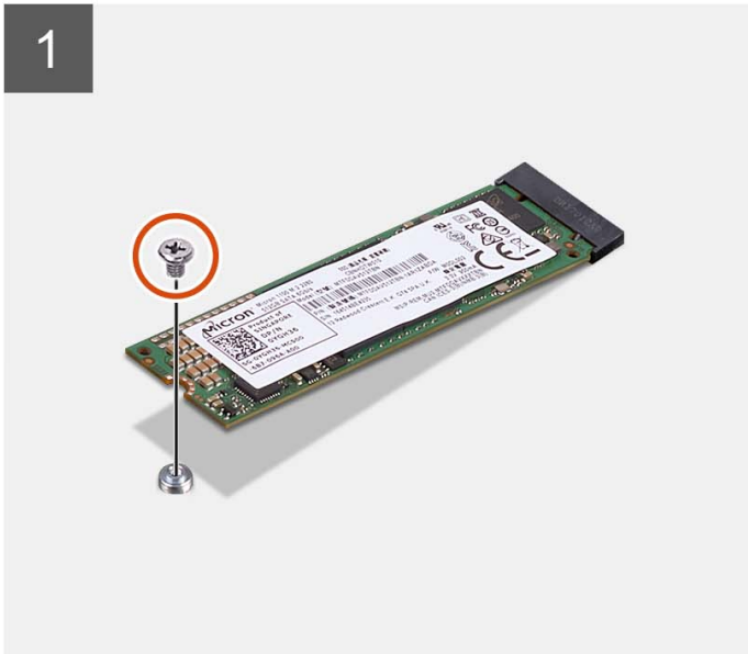
1x M2x3.5
